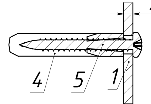
Б-Б 1 : 1
