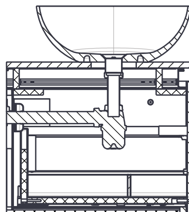
A-A (1:6)
