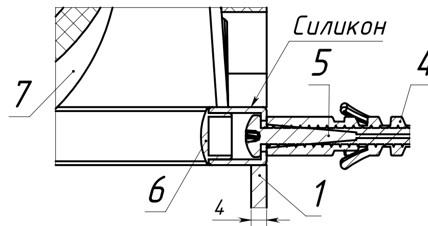
Б-Б 1 : 1
