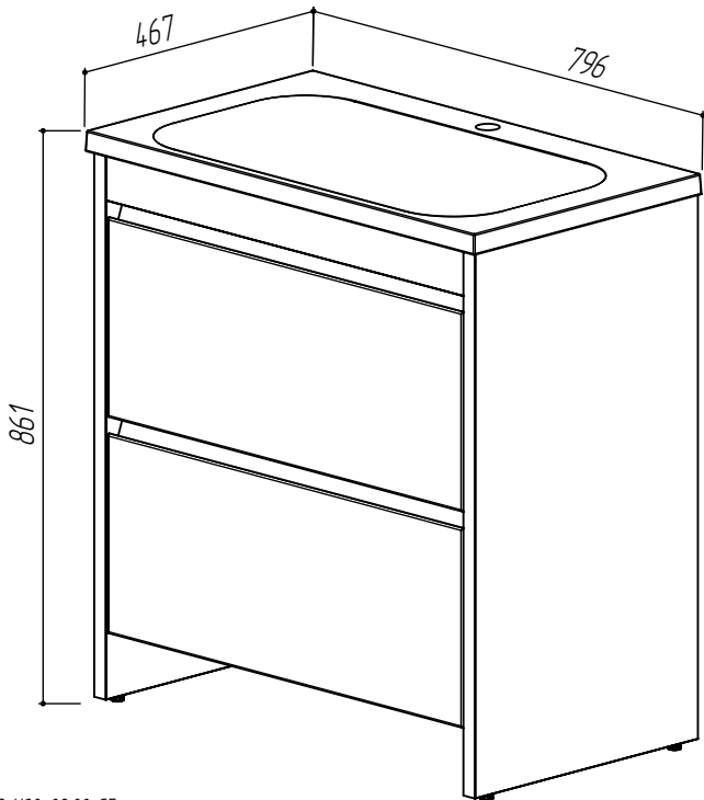
Модуль Н80-02.00 СБ
