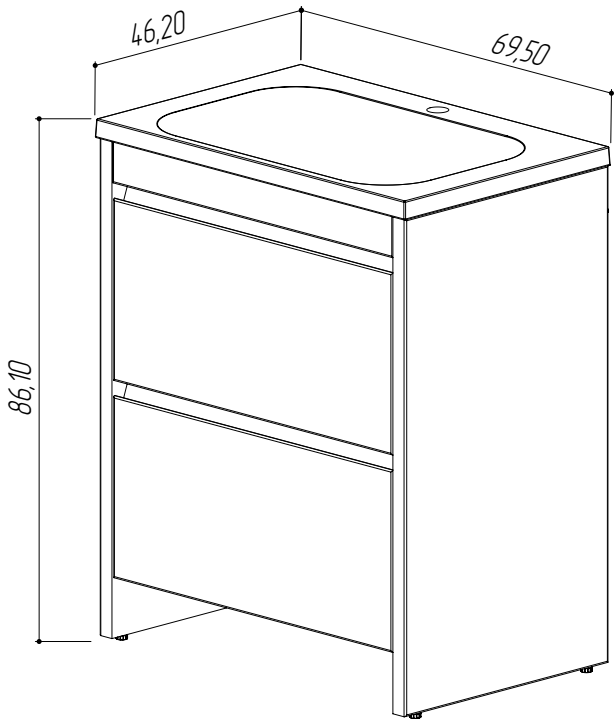
Модуль Н70-02.00 СБ
