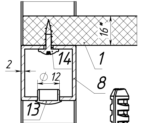
B-B 1 : 1
