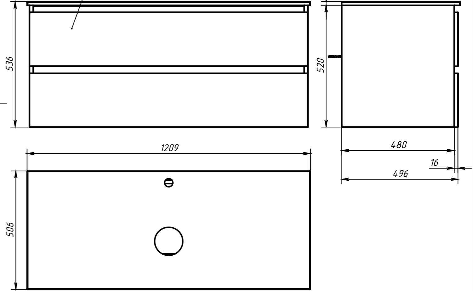
МОНБЛАН НП120-02.00 СБ
