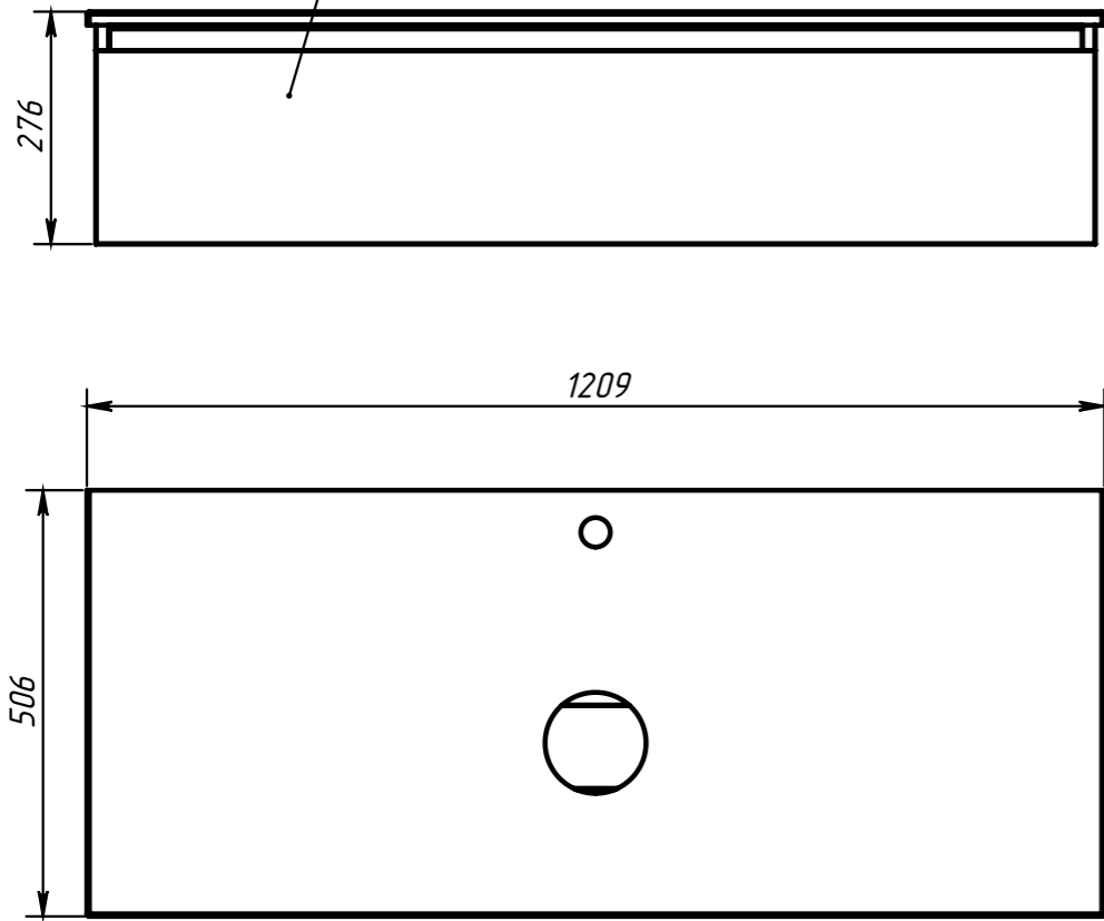
МОНБЛАН НП120-01.00 СБ
